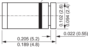
Glass MELF
